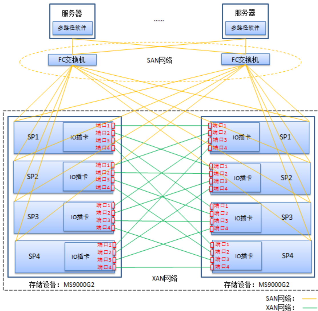
图4-3 四控 XAN 典型组网图（MESH 直连）
